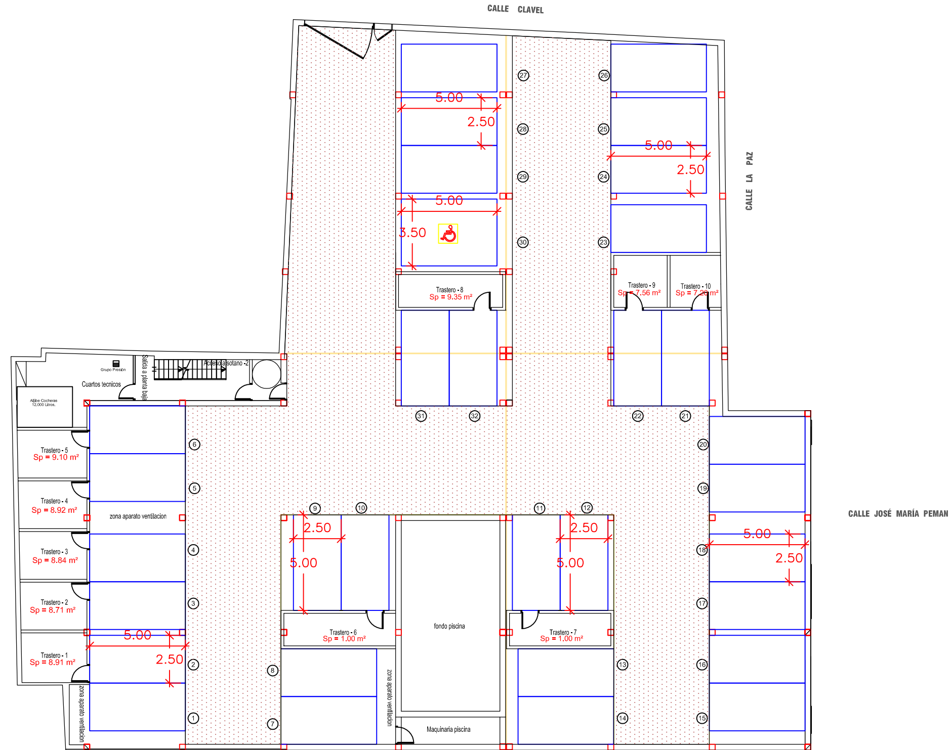
PLANTA SOTANO
